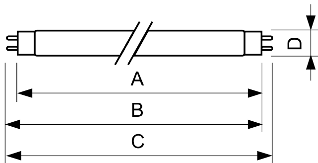
TL-D 36W/840
