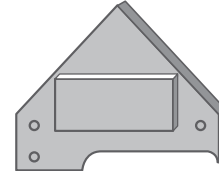
Door beam x1
